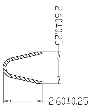
SEC:A-A
