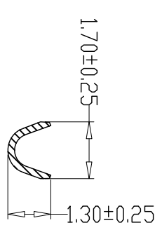
SEC:B-B
